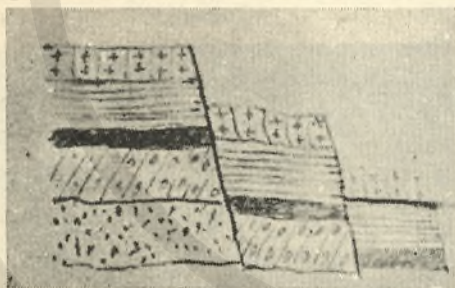
(Εἰκ. 20). Μονόπλευρος καθιζήσις.
