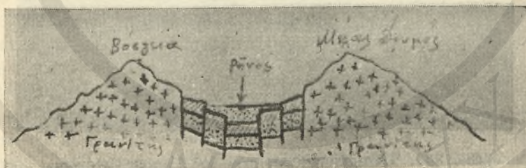
(Εἰκ. 22). Ταφροειδὴς ἐγκατακρήμνις σχηματίσασα τὴν κοιλάδα τοῦ Ρήνου.
