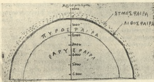
(Εἰκ 15). Τομή τῆς Γῆτινς Σφαίρας.
