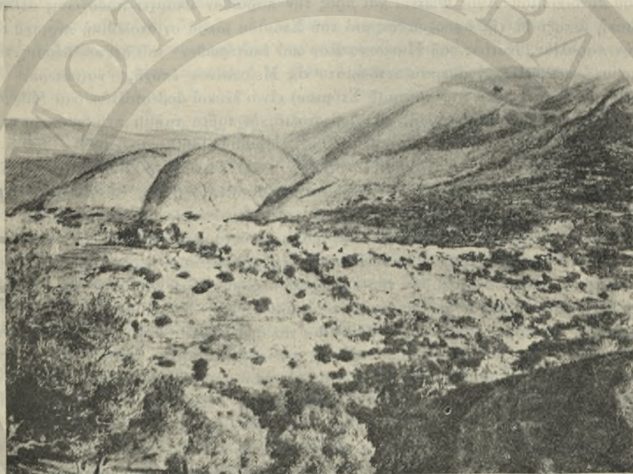
(Εἰκ. 5). Τὸ χωρίον Λάστρος ἐπὶ ἀσβεστολιθικοῦ τμήματος ἐν μέσῳ σχιστολιθικῶν πετρωμάτων.
