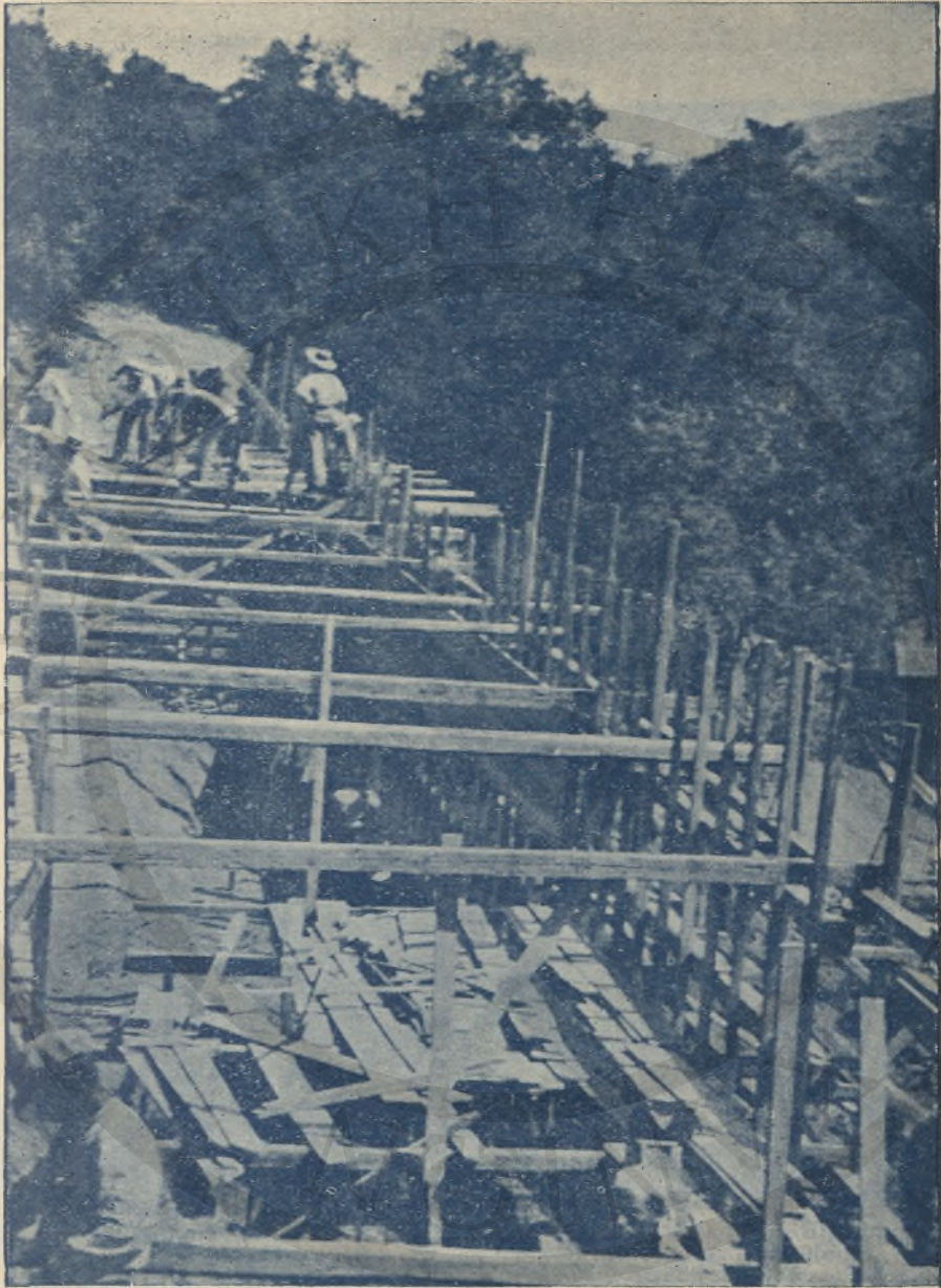
Υδραυλικά έργα Πλατανιά—Χανίων. Ξυλοτύπωσης πρὸς κατασκευὴν ἐκ βετοπ τμήματος τῆς κυρίας διώρυγος.
