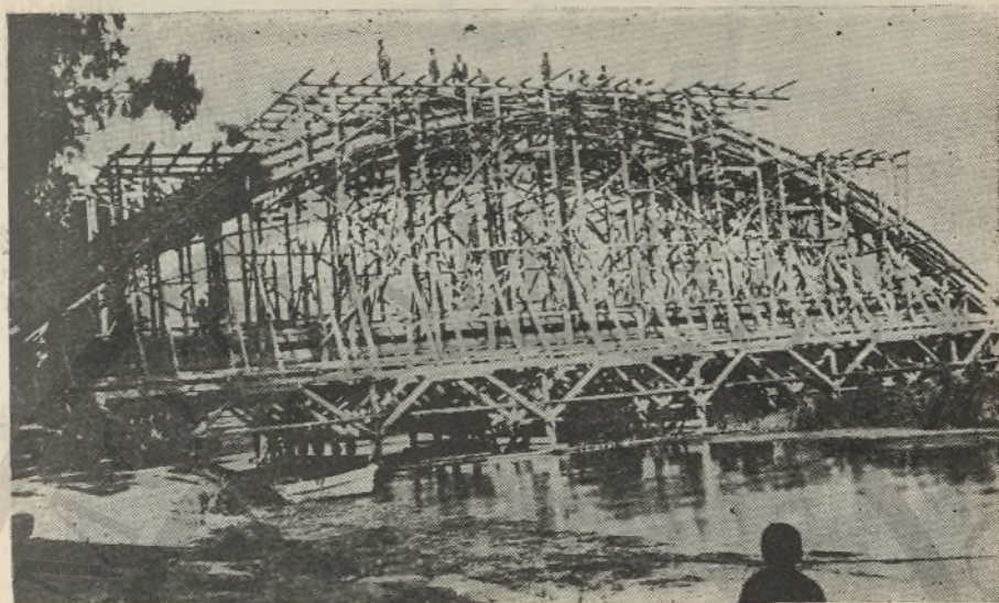
Ἡ ἀποπερατομένη γέφυρα Γεωργιουπόλεως Χανίων. «Ἴ. Μετιξᾶς» ἀνοίγματος 45 μ. ἧς ἡ δαπάνη ἀνήλθεν περί τὰ 2 ἑκατομ. δραχμῶν.
